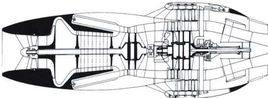
Projet d'un turboréacteur double flux à soufflante arrière SNECMA / RATEAU (1946) sur base du TA-1000
