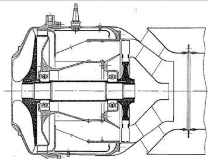
Turboréacteur de Sensaud de Laveau (1937)
