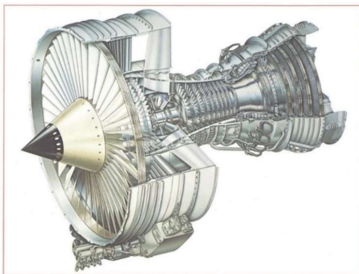
Ecorché du moteur CFM56-2
