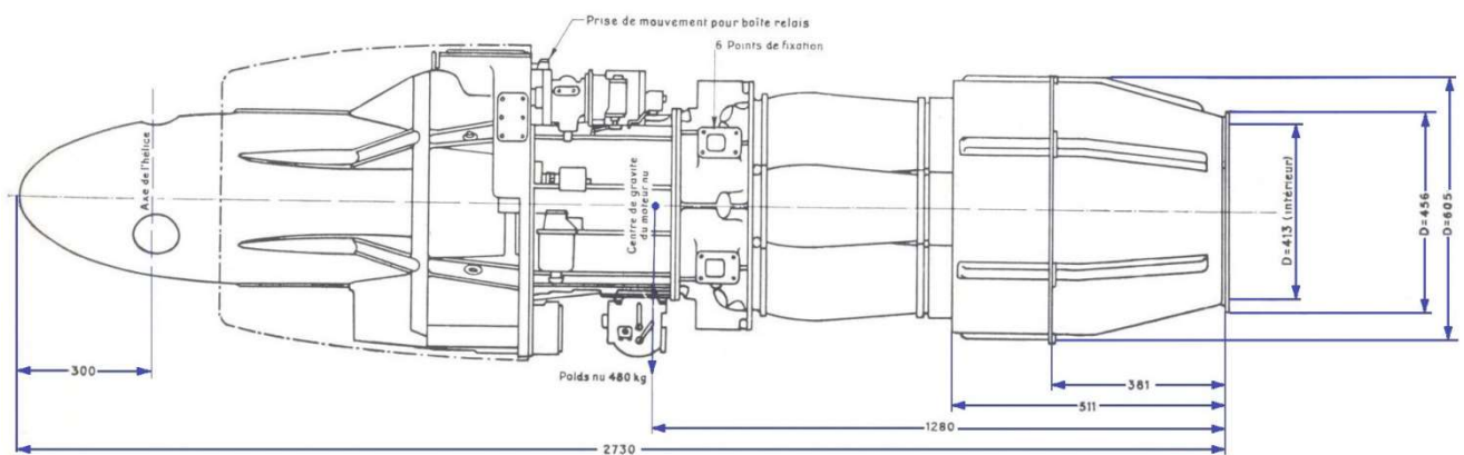
Coupe longitudinale du TB-1000
