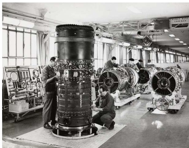
Chaîne de montage (Copyright Espace Patrimoine@Safran)
