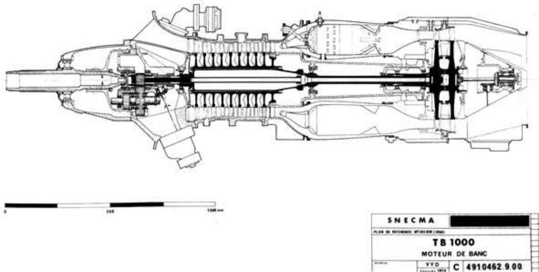
Coupe du TB-1000 - moteur de banc (1950) © Espace Patrimoine SAFRAN
