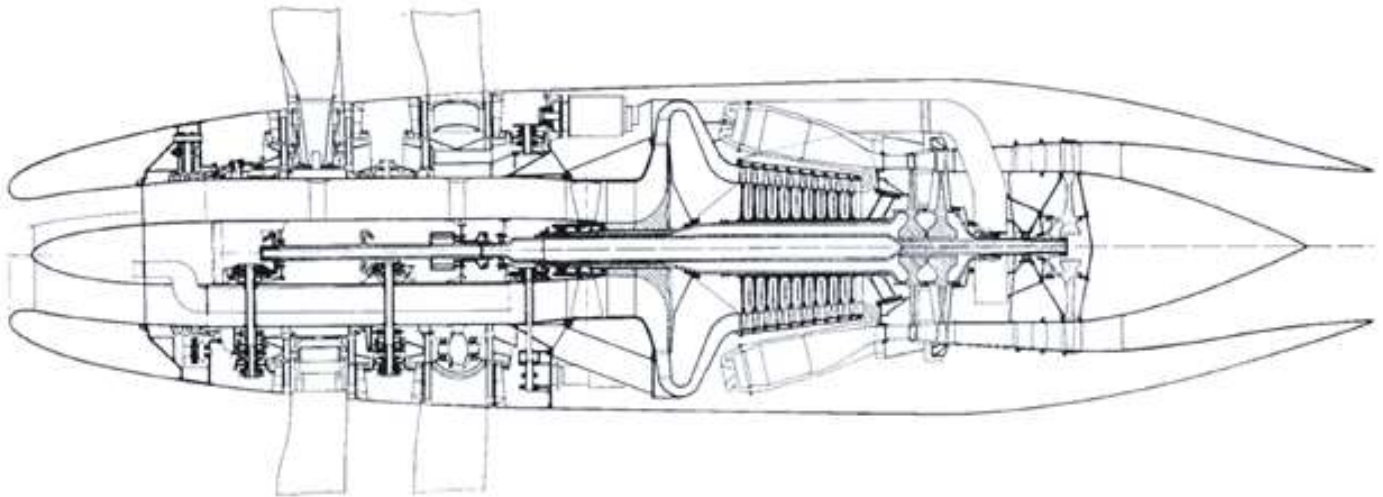
Coupe du turboréacteur SNECMA TA-1000
