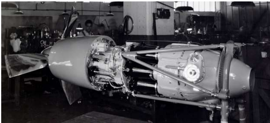
Le TB-1000 - © Espace Patrimoine Safran
