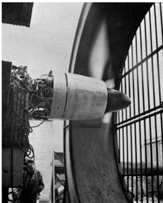
Le TB-1000 au banc d'essais à Villaroche- © Espace Patrimoine Safran
