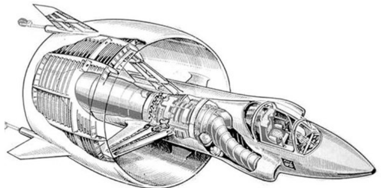
Ecorché C-450 Coléoptère surnommé "le char de Carnaval"
