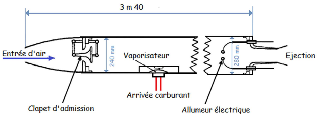
Projet de pulso-réacteur de Monsieur Charles de Louvrié (1867)
