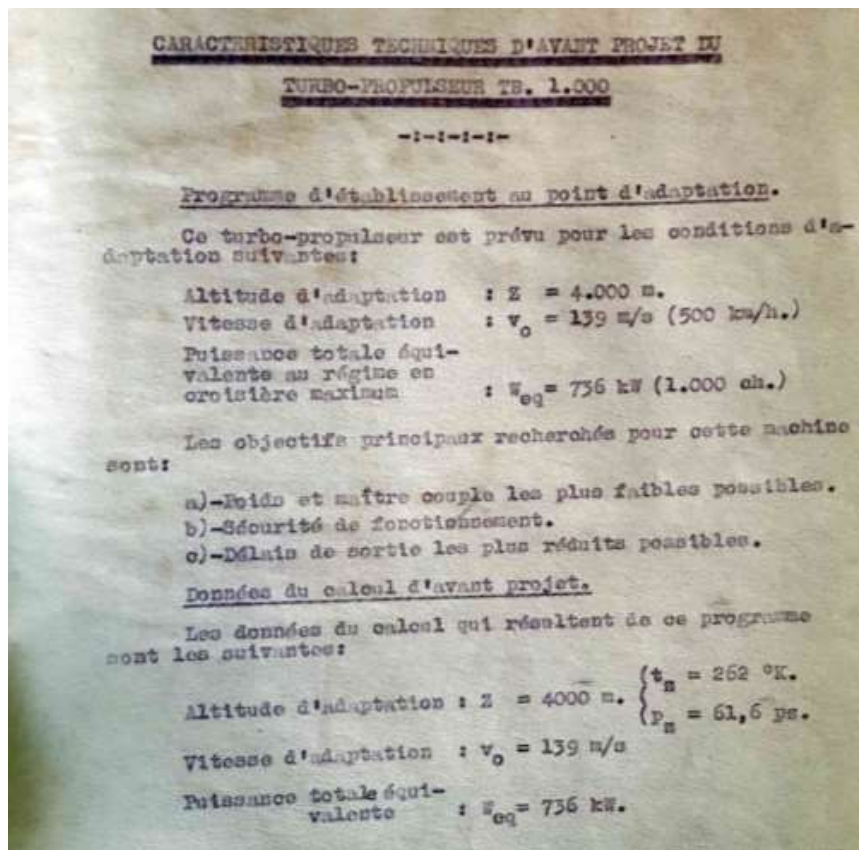
Les données générales techniques de l'avant-projet du TB-1000
