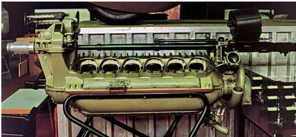
Canon HS 404 intégré au moteur H-S 12 Y (pour avions D-520 et M-S 406)
