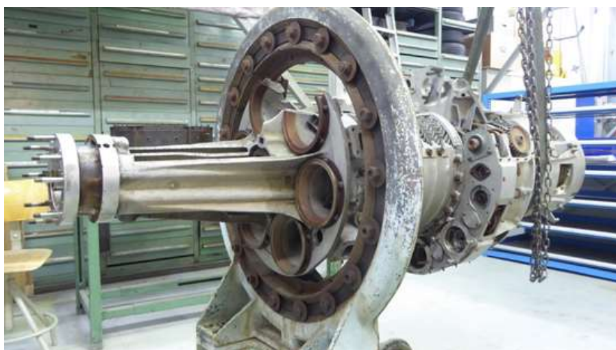
Après démontage complet des tubes à flamme de la chambre de combustion - 17/04/2019
