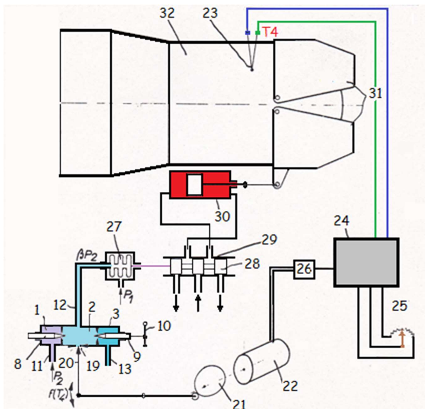
Croquis accompagnant le brevet de Mr Steiglitz
