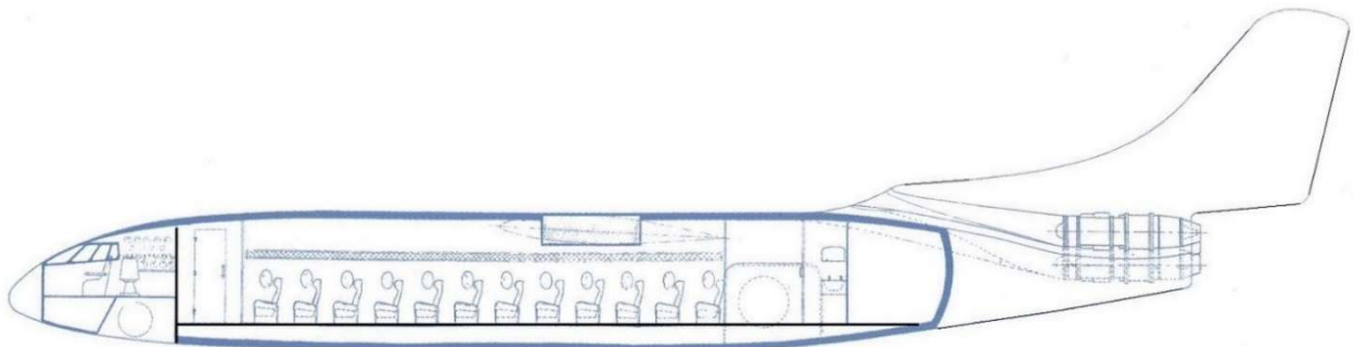
Avant-projet X210.02.10 avec trois Atar 101 alimentés par une entrée d'air unique (Juillet 1951)
