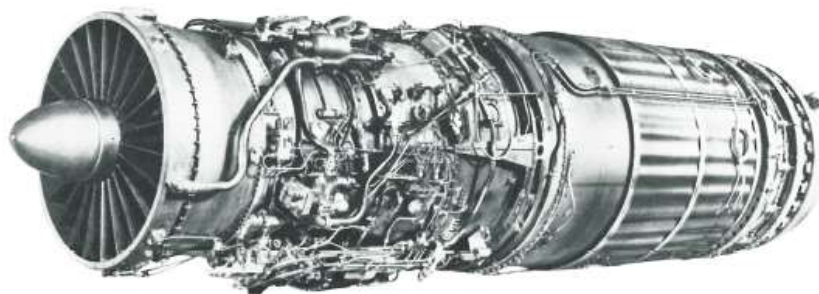
Turboréacteur double corps double flux TF-106 A (Copyright Espace Patrimoine Safran)
