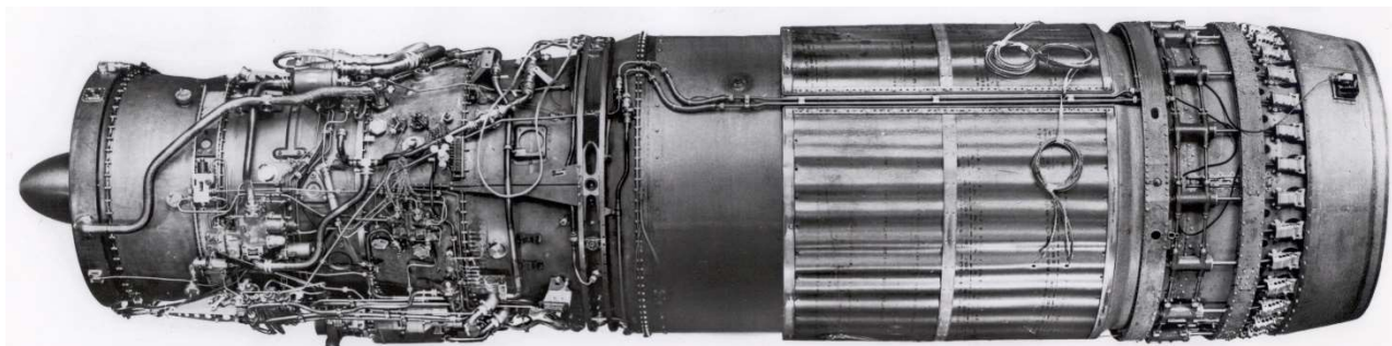
Turboréacteur double corps double flux TF-104 B (Copyright Espace Patrimoine Safran)
