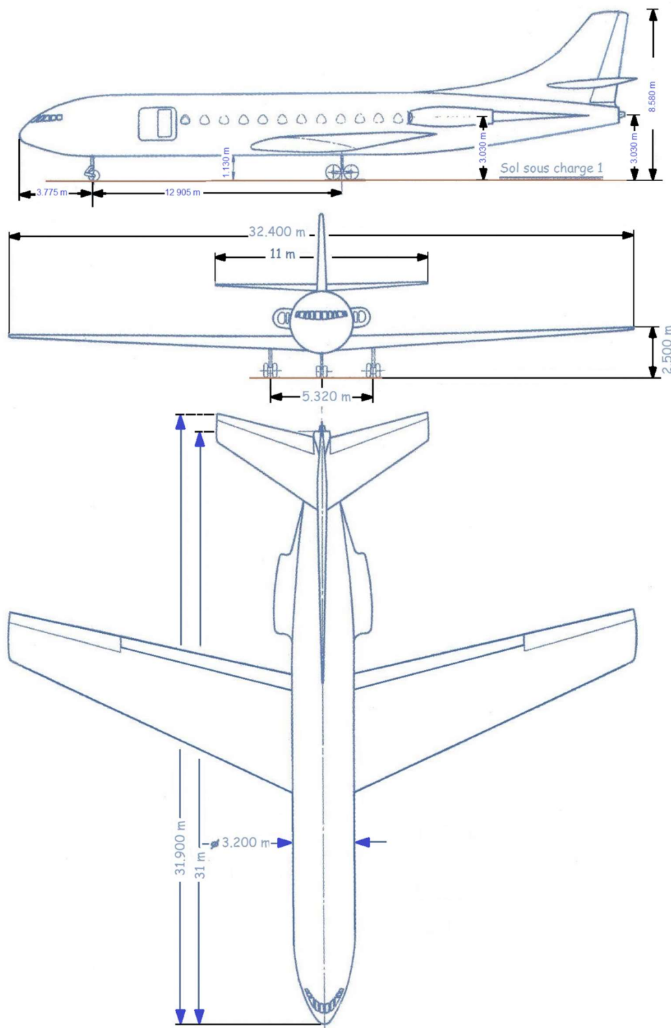
Plan trois vues de l'avant-projet X210.02.18 tri Atar 101 D (Décembre 1951)
