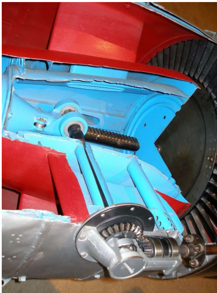
Commande de l'aiguille de tuyère du Jumo 004 - Photo P Mouton
