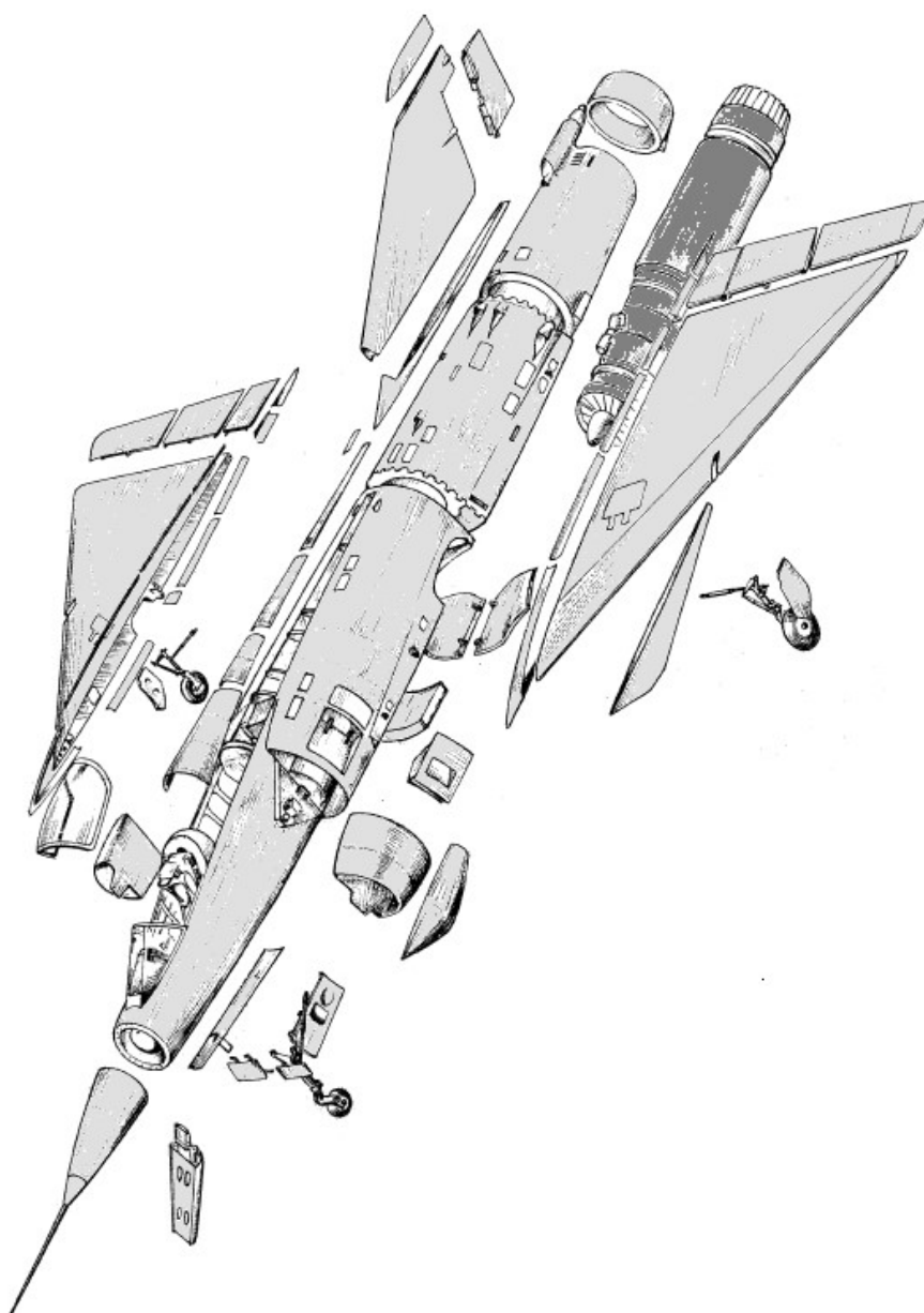
Mirage III T - Eclaté
