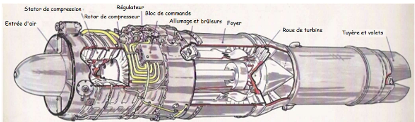
Snecma Atar 101 D
