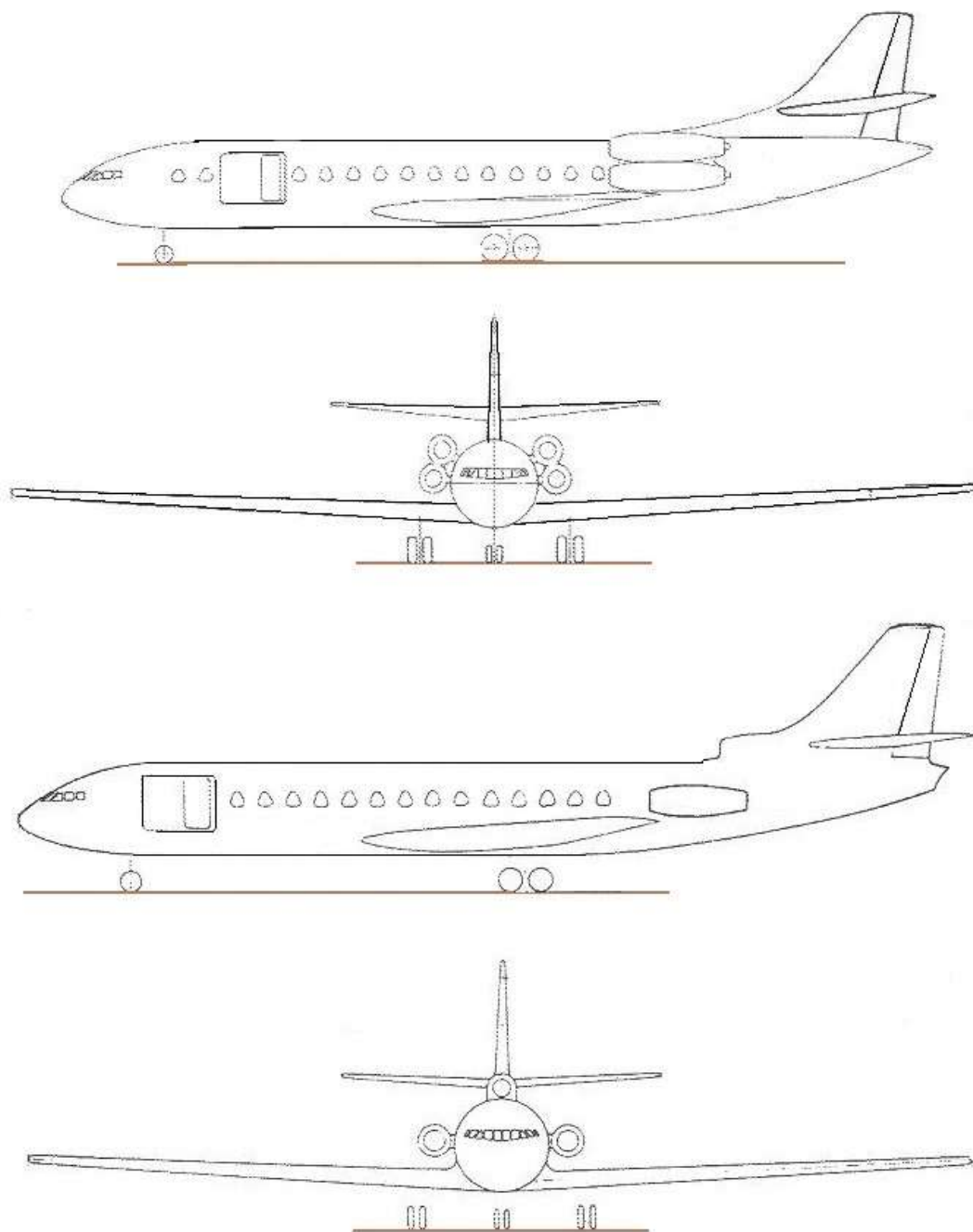
Plans des avant-projets X210.02.24 quadri Atar 101 D (mars 1952) et X210.02.28 tri Atar 101 D (mai 1952)
