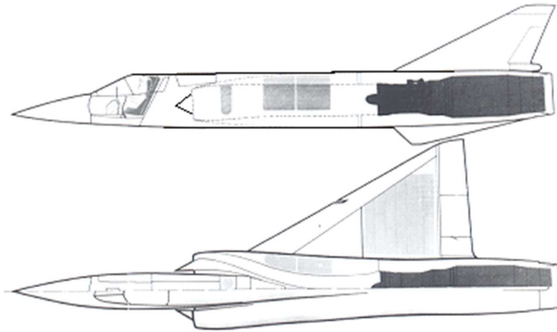
Mirage III T n° 01 : installation moteur
