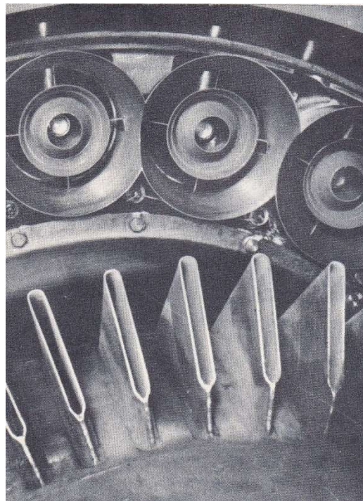
Détail de la chambre de combustion du BMW 003 - photo journal SNECMA
