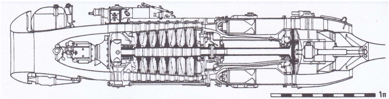
BMW 003 B - Coupe longitudinale
